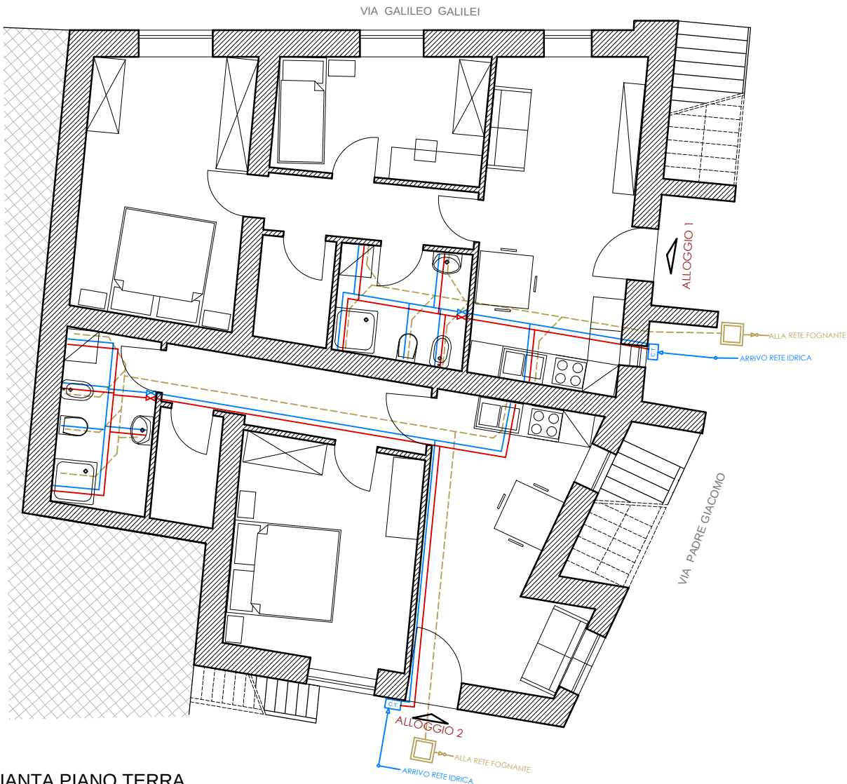
PIANTA PIANO TERRA Scala 1:50
