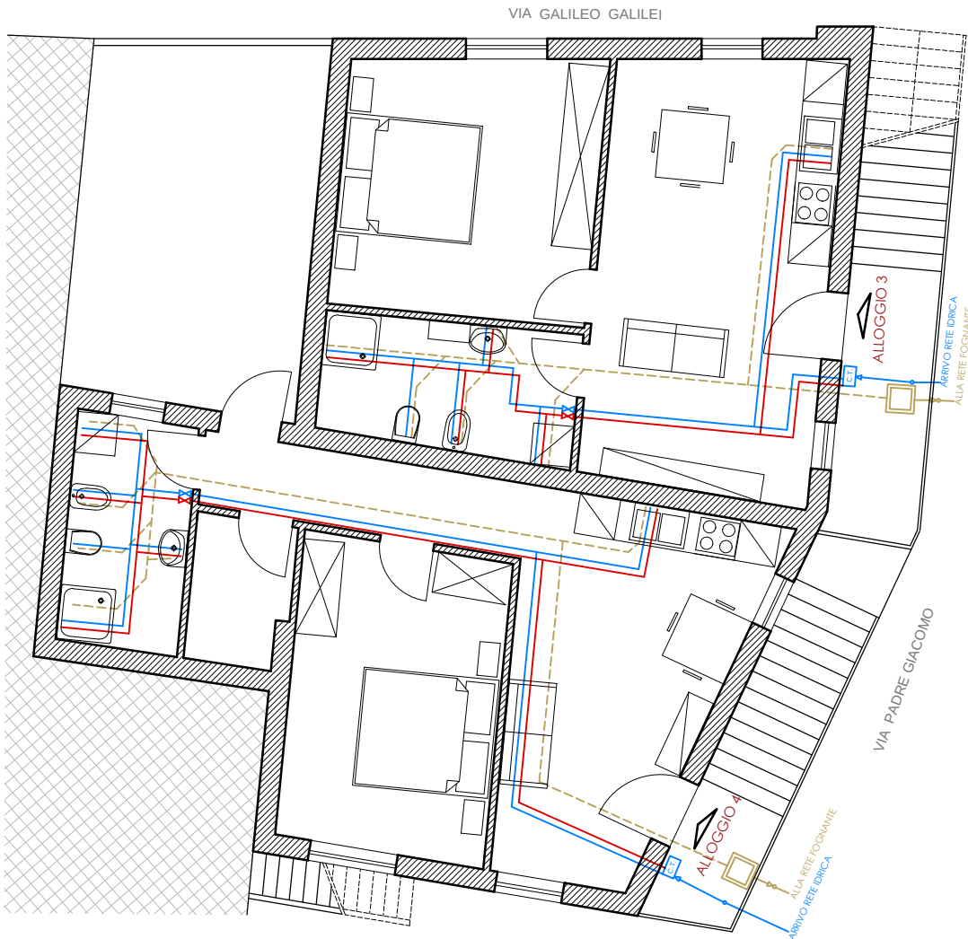
PIANTA PIANO PRIMO Scala 1:50
